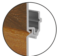
Détail A
